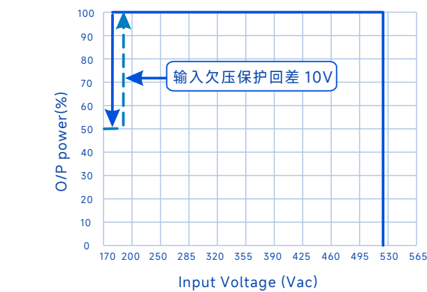
输出功率Vs.输入电压
